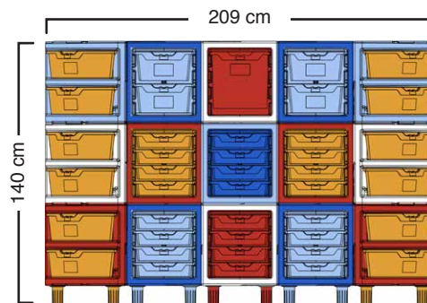
C008 3x3 + Cubeau angolare 3x3 + Corner Cubeau
