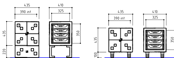
Cubeau con distanziali Cubeau with spacers
